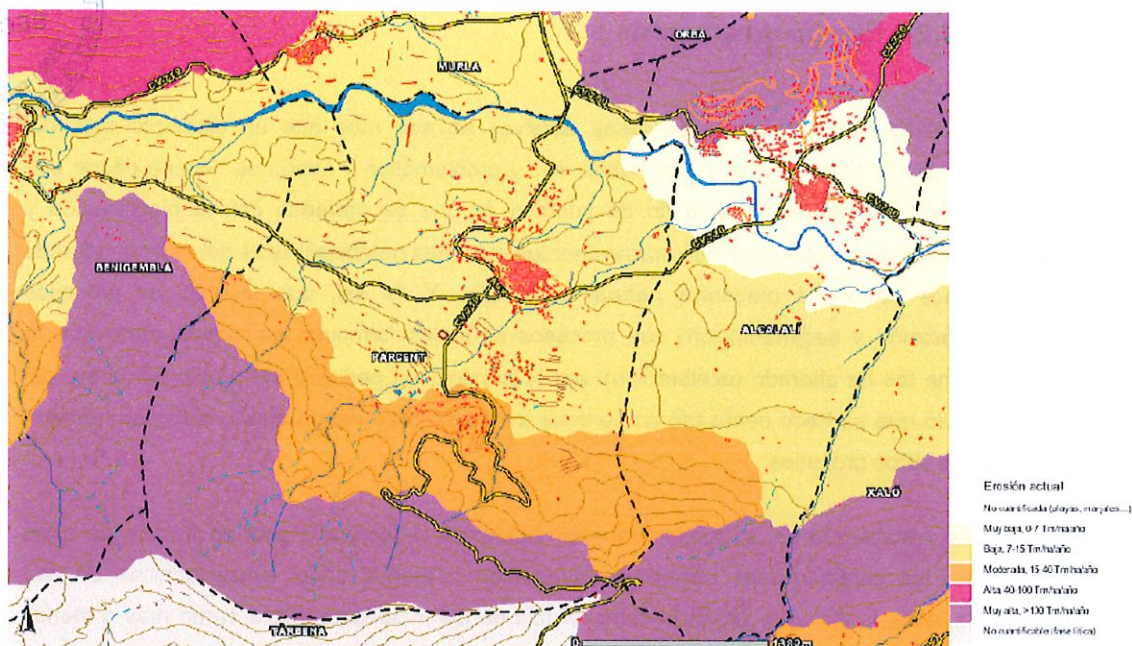
Riesgo de erosión actual (Conselleria de Medio Ambiente de la Comunitat Valenciana)
