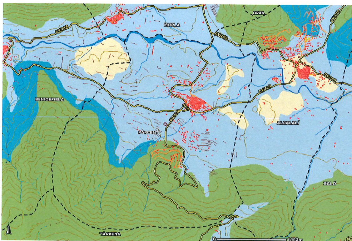
Vulnerabilidad de acuíferos
